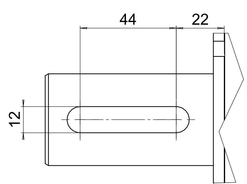
Optional Key: UNI 6607 A 12x8x56
